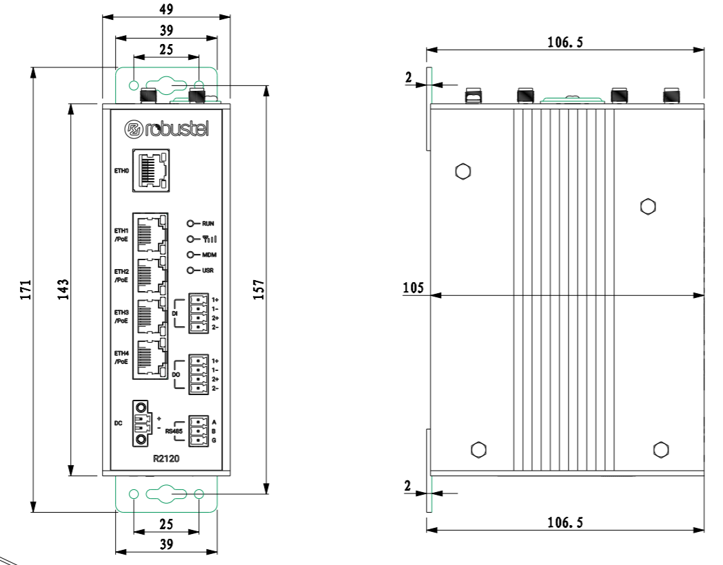
前视图 FRONT VIEW
