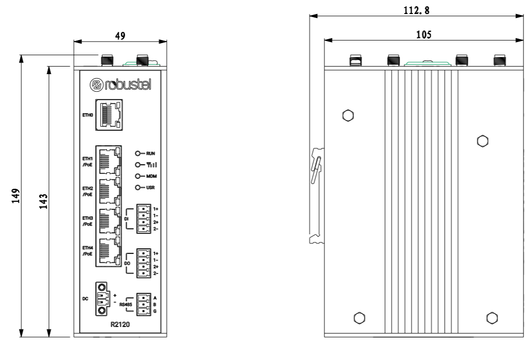
前视图 FRONT VIEW
